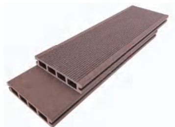
138H23-C 138*23 mm
